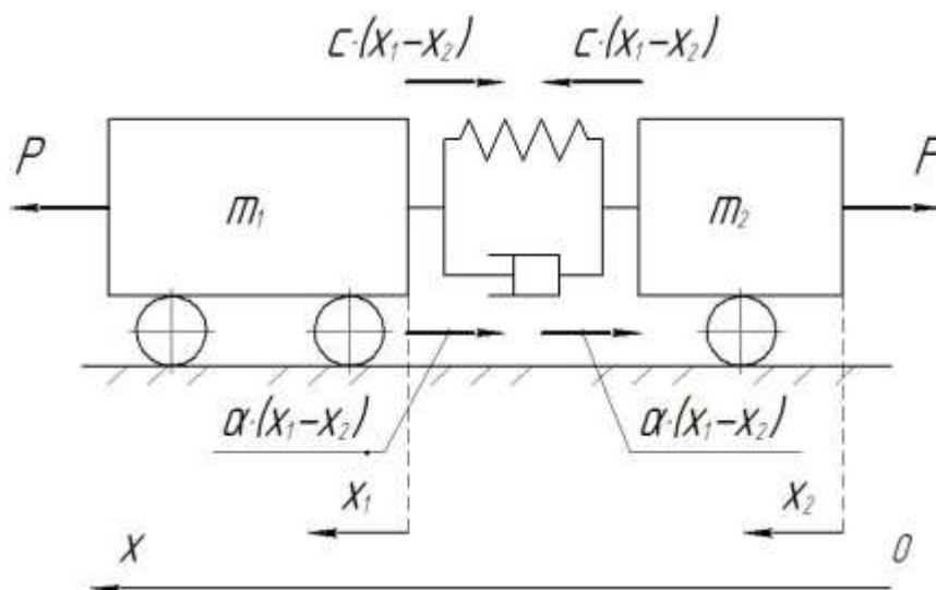
Рис. 1. Еквівалентна схема двохмасової системи «автомобіль – причіп»
